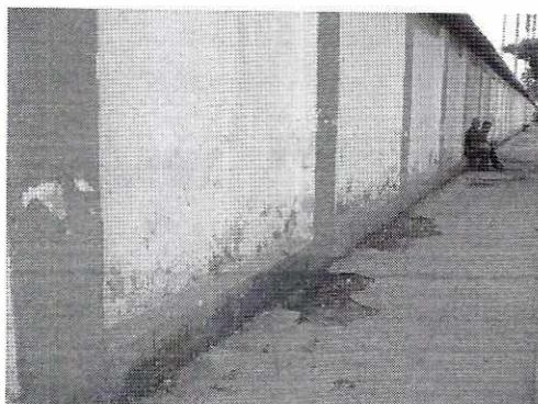
Foto 06- Detalhe do passeio apresentando falta de piso e parede externa com manchas por umidade e desprendimento da pintura.
